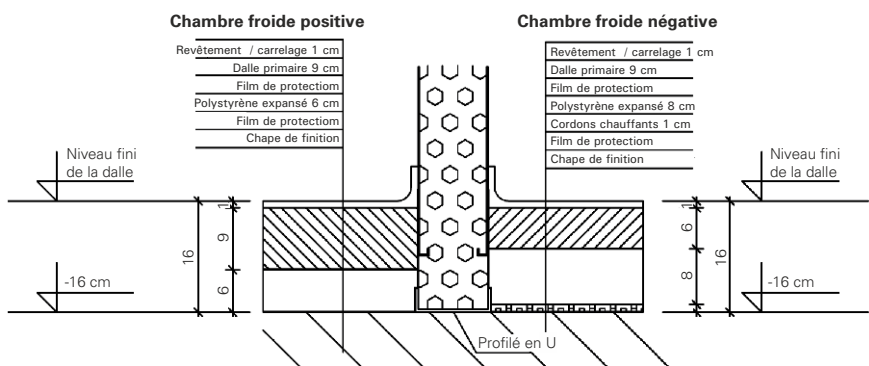
Schémat de la réalisation de l'isolation du plancher d'une chambre froide positive et négative
