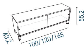
2 portes coulissantes Altuglas®
